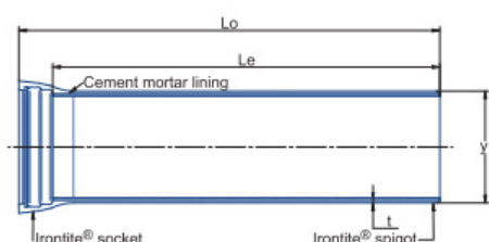
PN35 Irontite DI pipe spigot x socket
